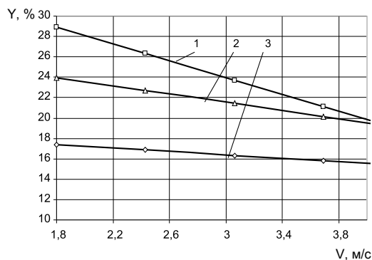
Рис. 2. Графіки залежностей впливу швидкості повітряного потоку на значення проходу стеблових матеріалів крізь сепаруючі поверхні при h = 9 мм: 1 — сепаруюча поверхня жалюзійного типу; 2 — сепаруюча поверхня жалюзійного типу зі струнами; 3 — сепаруюча поверхня комбінованого типу
