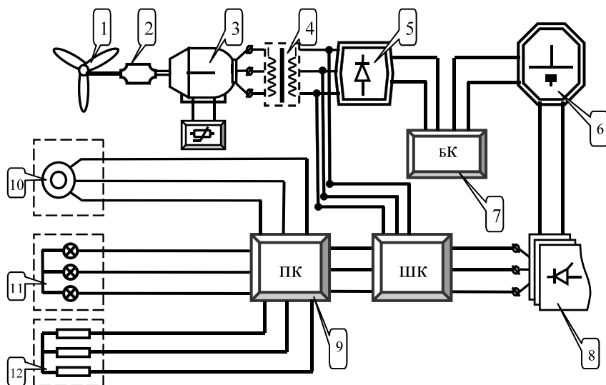
Рис. 4. Вітроенергетичний комплекс
