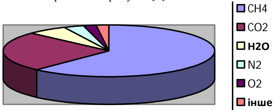
Рис.1. Склад біогазу
