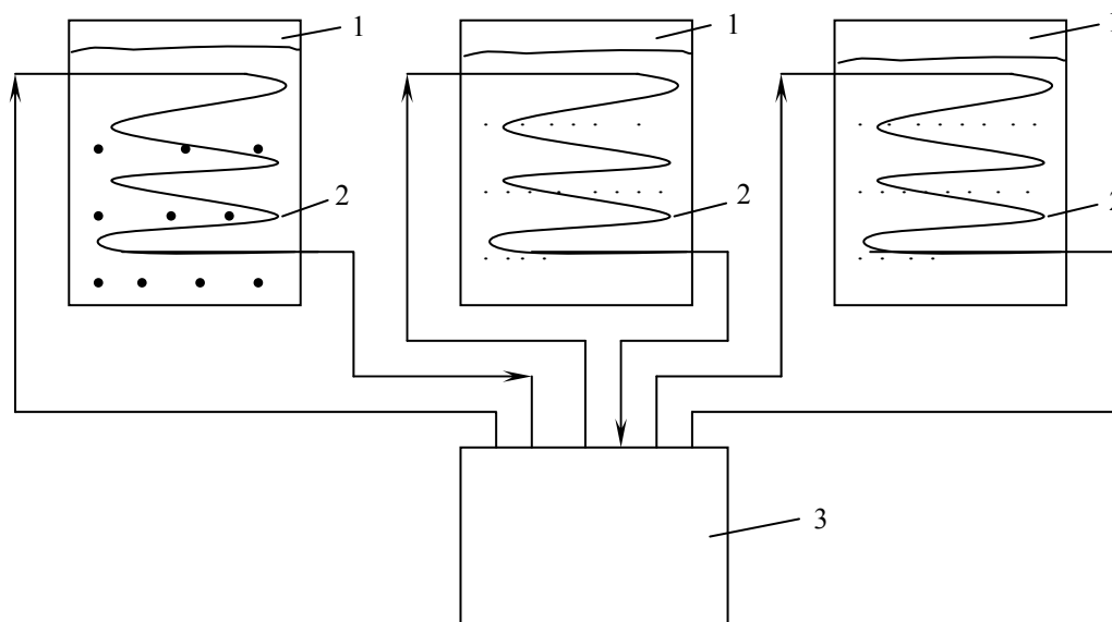
Рис. 1. Схема охлаждения зерна при помощи стационарной холодильной машины
