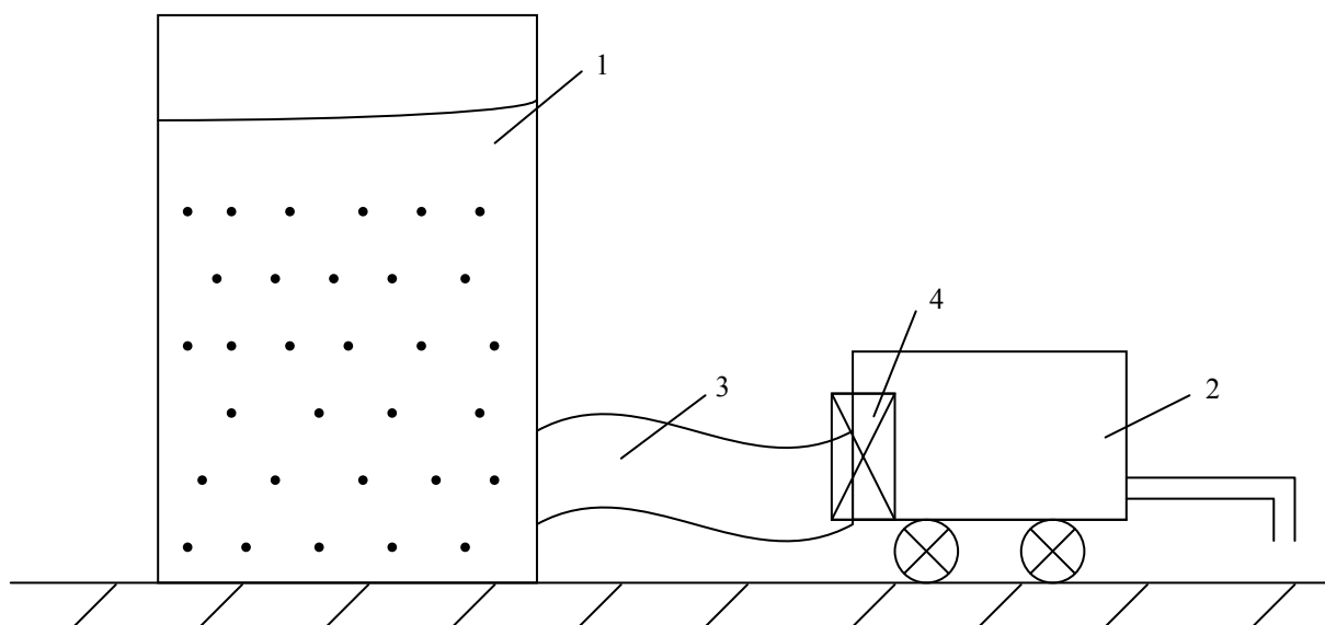
Рис. 2. Схема охлаждения зерна с помощью мобильной холодильной машины
